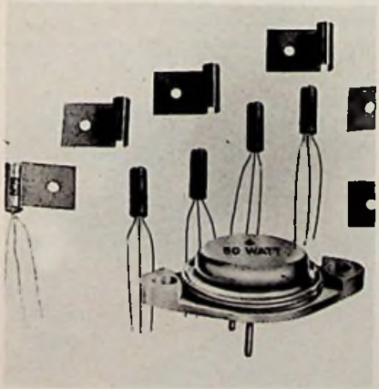
Afb. 2. Het reeds vergrijsde germanium vermogenswerk... naast een huidige krachtpatser.
